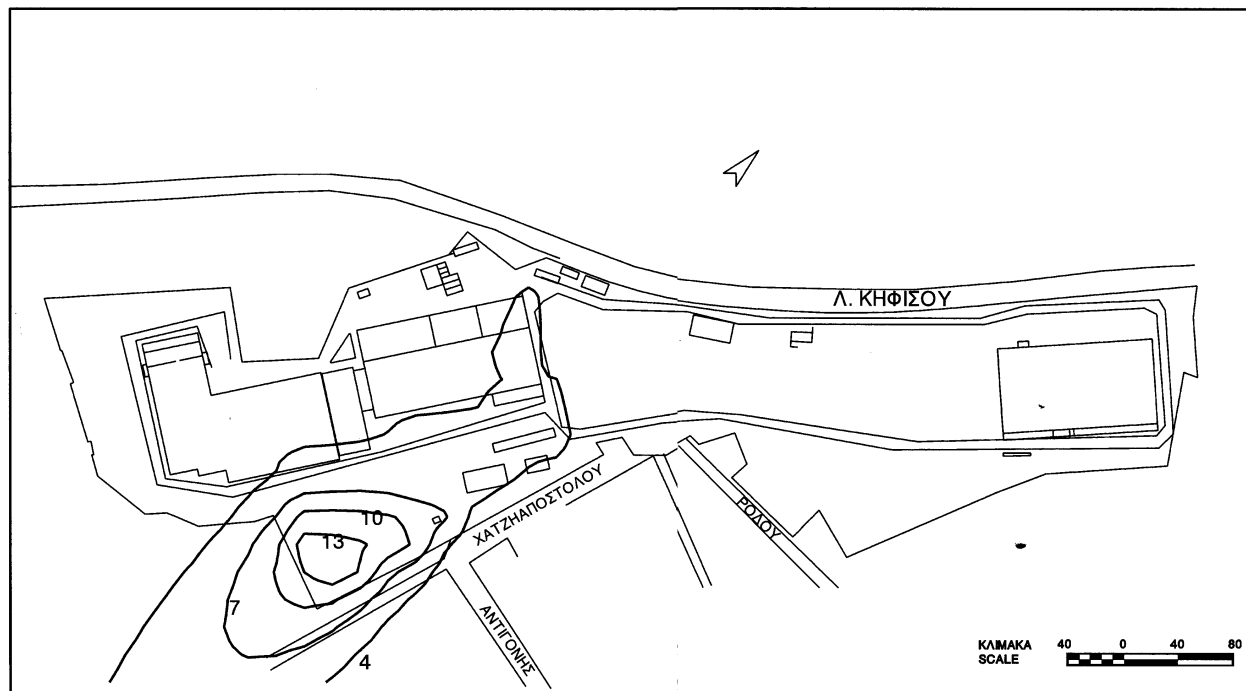
ΣΧΗΜΑ II.7 Ισοσυγκεντρωσιακές καμπύλες Δραστηριότητες Αμαξοστασίου Σεπολίων Ρύπος CO (σε \mu\text{g}/\text{m}^3 ), Έτος 2018
