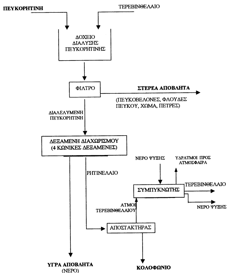
ΔΙΑΓΡΑΜΜΑ ΡΟΗΣ ΠΑΡΑΓΩΓΙΚΗΣ ΔΙΑΔΙΚΑΣΙΑΣ ΕΠΕΞΕΡΓΑΣΙΑΣ ΠΕΥΚΟΡΗΤΙΝΗΣ
