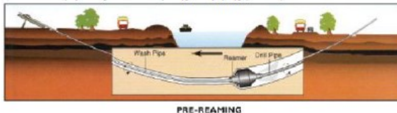
Διαδικασία Οριζόντιας Κατευθυνόμενης Διάτρησης (H.D.D.)
