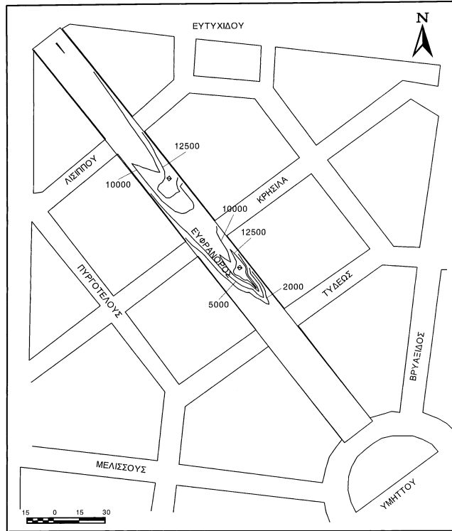
ΜΕΛΕΤΗ ΠΕΡΙΒΑΛΛΟΝΤΙΚΩΝ ΕΠΙΠΤΩΣΕΩΝ ΥΠΟΓΕΙΟΥ ΣΤΑΘΜΟΥ ΑΥΤΟΚΙΝΗΤΩΝ ΠΛΑΤΕΙΑΣ ΕΥΦΡΑΝΟΡΟΣ ΙΣΟΣΥΓΚΕΝΤΡΩΤΙΚΕΣ ΚΑΜΠΥΛΕΣ (µg/m 3 ) ΤΟΥ ΡΥΠΟΥ CO που οφείλεται στη λειτουργία του σταθµού. ΑΤΜΟΣΦΑΙΡΙΚΗ ΡΥΠΑΝΣΗ ΚΑΤΑ ΤΗ ΛΕΙΤΟΥΡΓΙΑ ΤΟΥ ΕΡΓΟΥ
