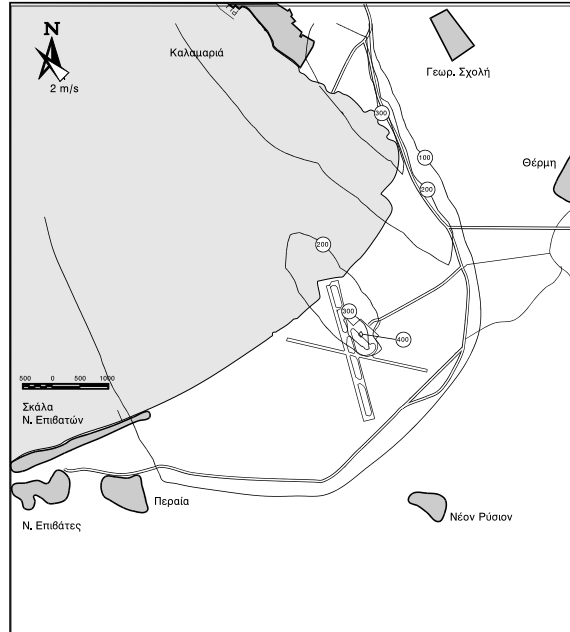
ΑΠΟΤΕΛΕΣΜΑΤΑ ΡΕΥΣΤΟΔΥΝΑΜΙΚΟΥ ΜΟΝΤΕΛΟΥ ΙΣΟΣΥΓΚΕΝΤΡΩΤΙΚΕΣ ΚΑΜΠΥΛΕΣ (µg/m 3 ) ΣΕΝΑΡΙΟ ΜΕ ΕΡΓΑ ΕΤΟΣ : 1997 ΡΥΠΟΣ : CO
