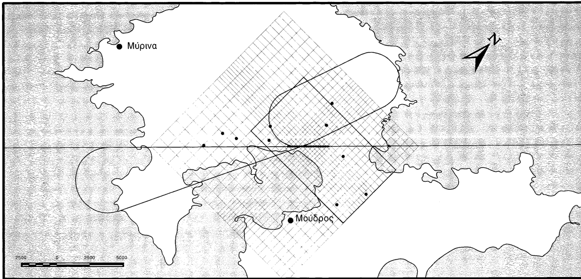
ΥΠΟΛΟΓΙΣΤΙΚΟ ΠΛΕΓΜΑ Ευρύτερη περιοχή εφαρμογής του Ρευστοδυναμικού μοντέλου όπου φαίνονται και οι διαδρομές των Α/Φ κατά την απογείωση και προσγείωση
