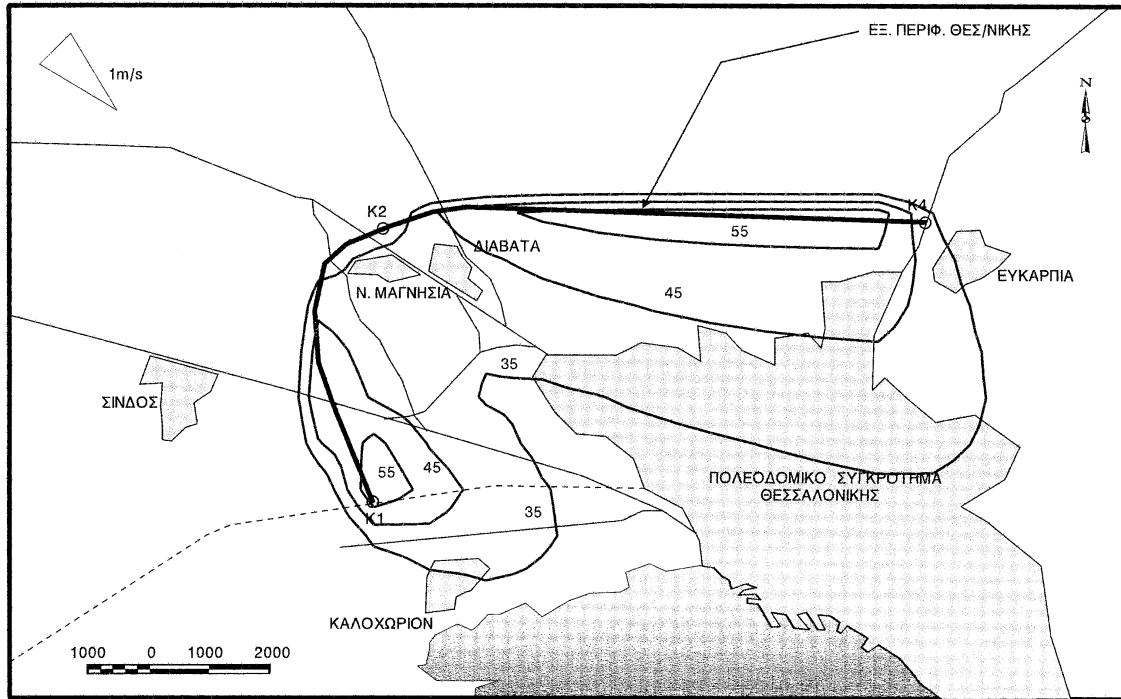
ΙΣΟΣΥΓΚΕΝΤΡΩΤΙΚΕΣ ΚΑΜΠΥΛΕΣ (µg/m 3 ) ΤΟΥ ΡΥΠΟΥ ΝΟ x ΕΤΟΣ 2011. ΕΞΩΤΕΡΙΚΗ ΠΕΡΙΦΕΡΕΙΑΚΗ ΘΕΣΣΑΛΟΝΙΚΗΣ
