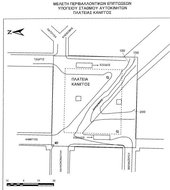
ΙΣΟΣΥΓΚΕΝΤΡΩΤΙΚΕΣ ΚΑΜΠΥΛΕΣ (µg/m 3 ) ΤΟΥ ΡΥΠΟΥ NO x ΥΦΙΣΤΑΜΕΝΗ ΚΑΤΑΣΤΑΣΗ
