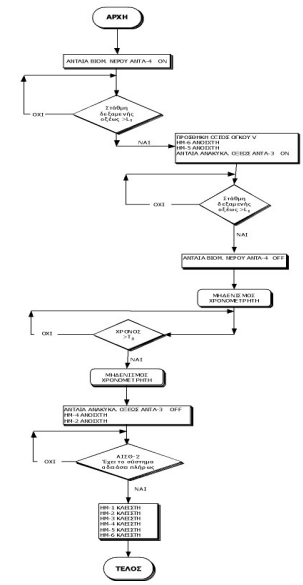
ΠΑΥΣΙΜΟ ΜΕ ΟΞΥ ΚΑΙ ΑΔΕΙΑΣΜΑ ΔΕΞΑΜΕΝΗΣ ΟΞΕΩΣ
